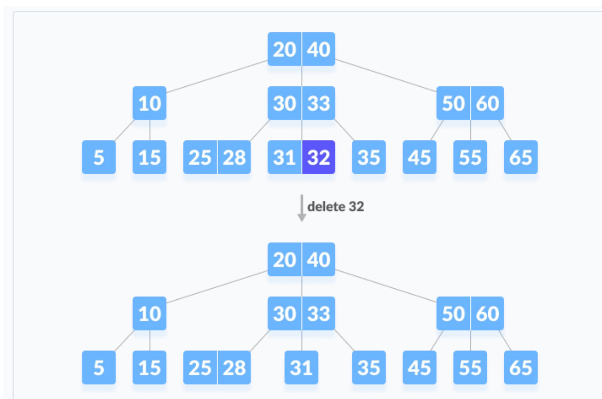
Figura 18: Árbol B
