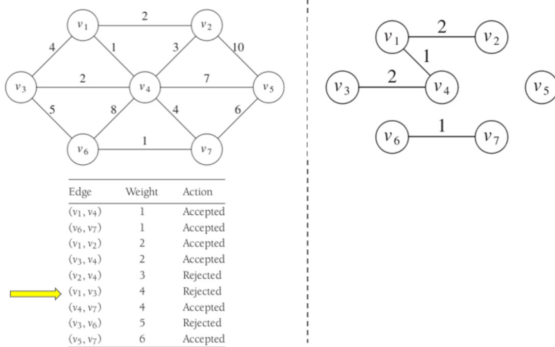
Figura 55: Kruskal
